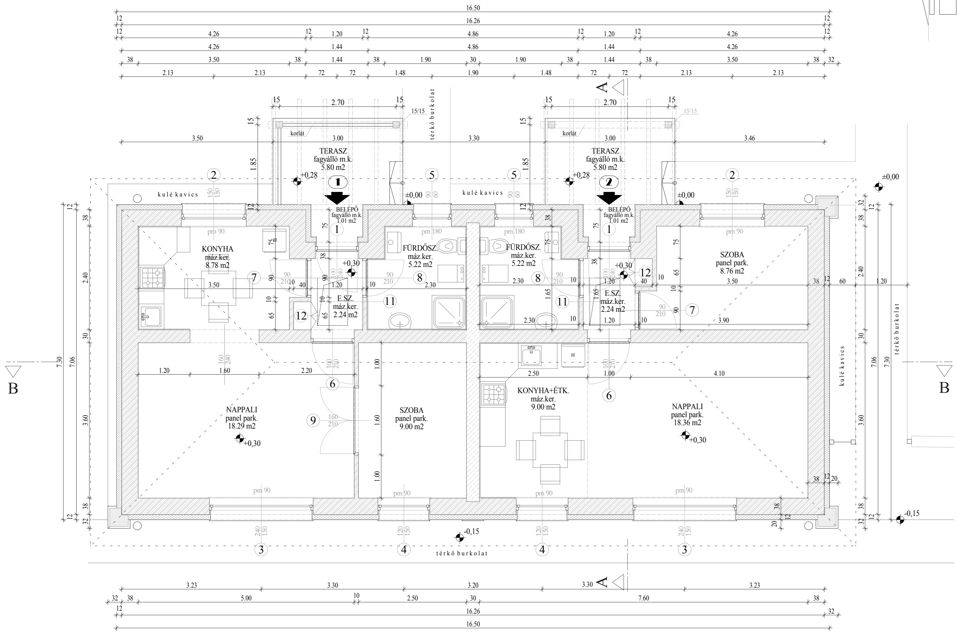
ALAPRAJZ, M:150
